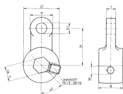
For funksjonsoverføring fra det ene hjelparet til det andre
