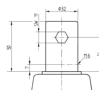
For montering av egenprodusert pedal av rør
